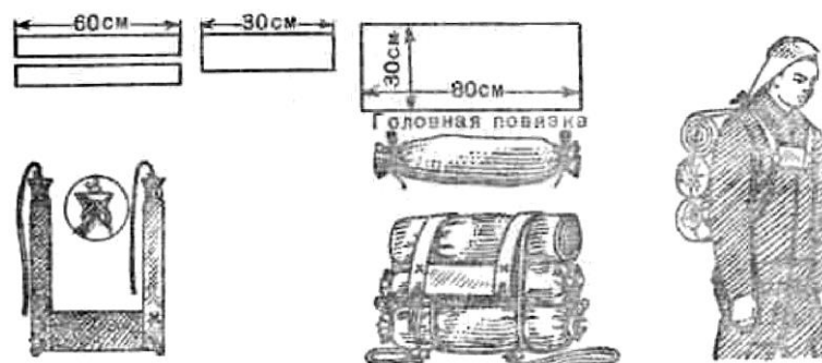
Рис. 31. Изготовление вещевого мешка из подручных материалов Для грудного и плечевого ремней используйте лямки парашюта. Привяжите или пришейте стропу к лямкам, как показано на рисунке. Сделайте петли из строп. Предметы для переноски заверните в парашютную ткань в виде двух скаток. Сделайте петли на обеих стропках нижней скатки для присоединения к лямке. Скатки свяжите вместе стропой
